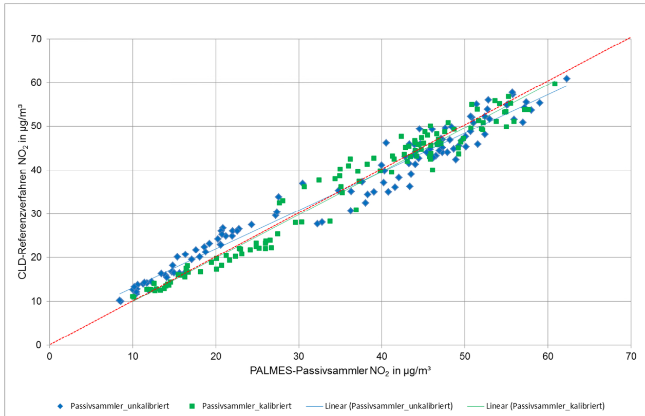
Abb. 1: Vergleich unkalibrierter und kalibrierter \text{NO}_2 -Passivsammlerdaten dem Referenzverfahren
